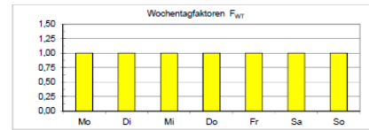
Wochentagfaktoren F_{WT}
